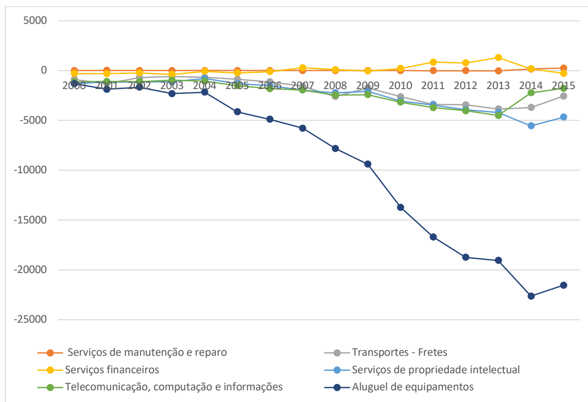
Gráfico 19. Balança de serviços por rubrica (Brasil - US$ milhões correntes)
